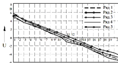
Рисунок 8 – Изменение выходного напряжения от электронного датчика шкворня в зависимости от прикладываемой силы
