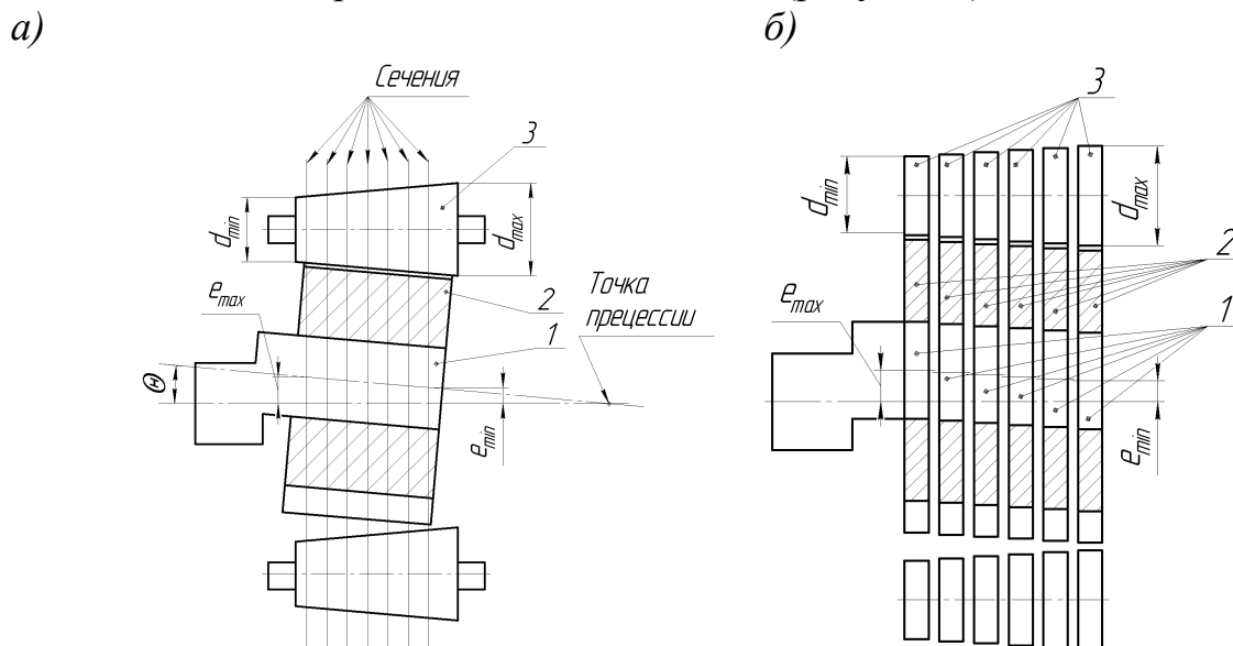
а – планетарная прецессионная передача с разбивкой ее по сечениям; б – набор тонкослойных сечений, составляющих планетарную прецессионную передачу; 1 – эксцентрик; 2 – сателлитное колесо; 3 – конический ролик
