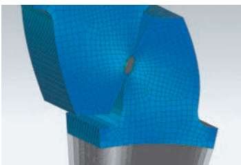
Конечно-элементная модель эвольвентного зацепления
