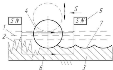
Рис. 1. Схема осуществления совмещенного МДН в активной технологической среде
