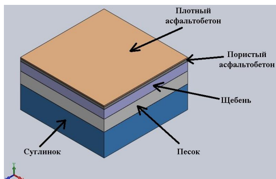
Рис. 3. Моделируемая конструкция дорожной одежды
