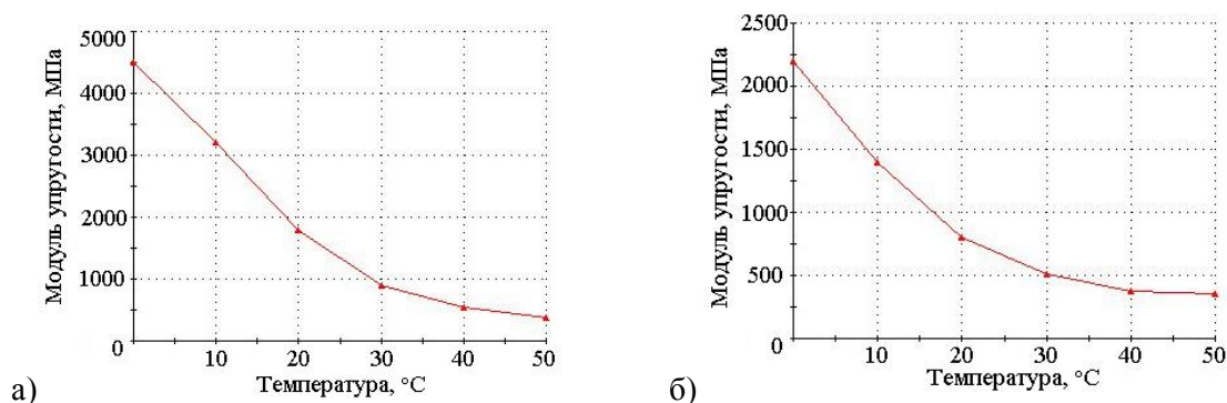
Рис. 2. Зависимость модуля упругости асфальтобетона от температуры а – для плотного асфальтобетона; б – для пористого асфальтобетона
