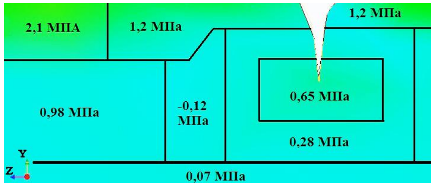
Рис. 7. Поле напряжений вблизи трещины шириной раскрытия 2 см и глубиной 2 см под воздействием температуры
