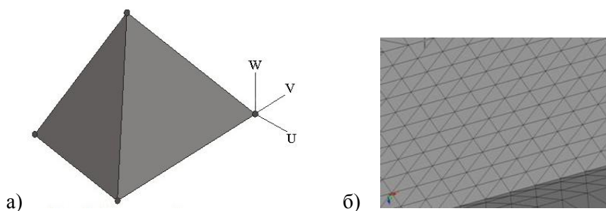
Рис. 1. К описанию сущности метода конечных элементов:
