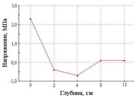
Рис. 6. Распределение напряжений при одновременном действии транспортной нагрузки и температуры
