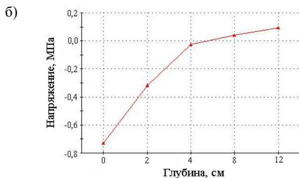
Рис. 5. Результаты моделирования для асфальтобетонных слоев покрытия
