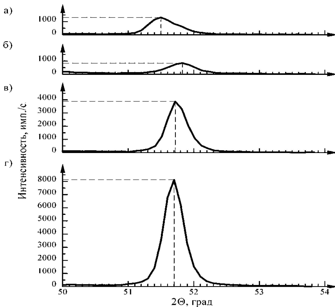
Рис. 7. Профиль линии (111) никеля: а – исходное состояние; б – после обработки с удельной мощностью горения разряда 0,20 кВт/м 2 ; в – после обработки с удельной мощностью горения разряда 0,50 кВт/м 2 ; г – после обработки с удельной мощностью горения разряда 0,88 кВт/м 2
