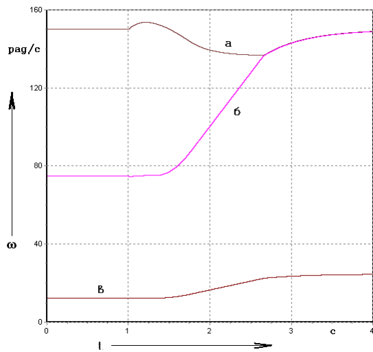
а) угловая скорость ведущего вала; б) угловая скорость ведомого вала; в) угловая скорость выходного вала; Рисунок 8 - Изменение угловых скоростей в коробке передач при переключении ступеней
