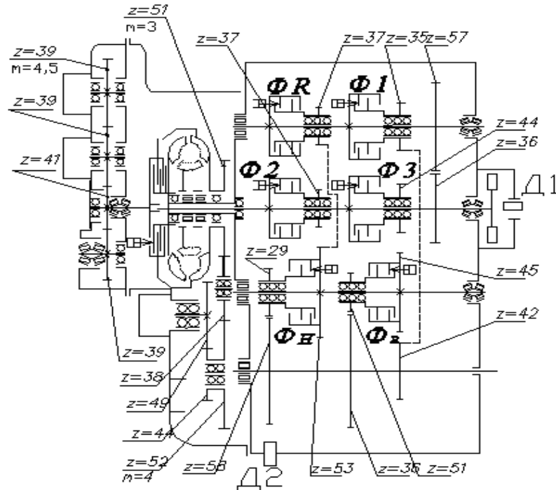
Рис. 3 - Схема установки импульсных датчиков на ГМКП БелАЗ-7555.
