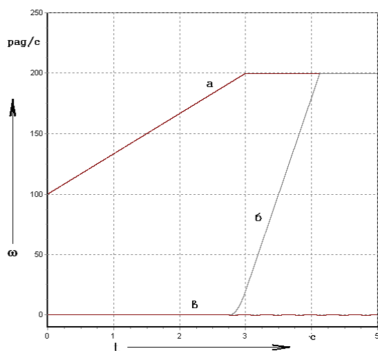
а) угловая скорость двигателя; б) скорость турбинного вала; в) скорость выходного вала; Рис.6 –Графики угловых скоростей при диагностировании фрикциона
