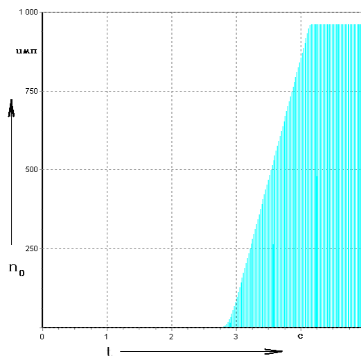
Рис.7 – Определение наличия буксования фрикциона импульсной системой в стоповом режиме
